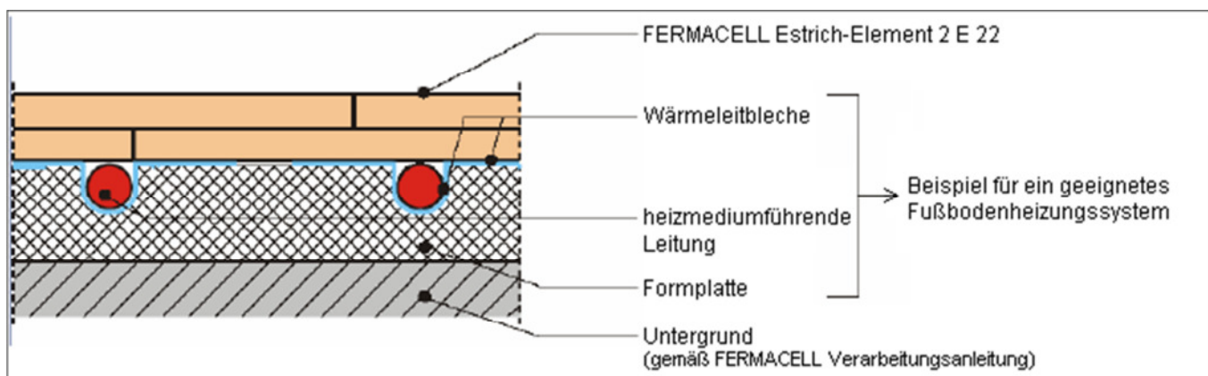
Aufbau Fermacell Estrich-Element (25 mm) mit Fußbodenheizungssystem
